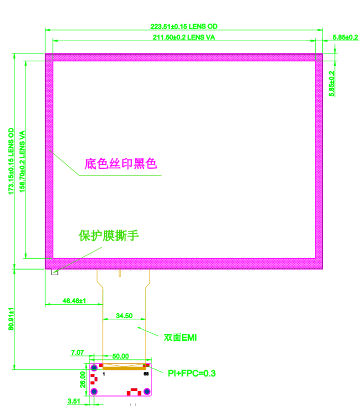
正视图
