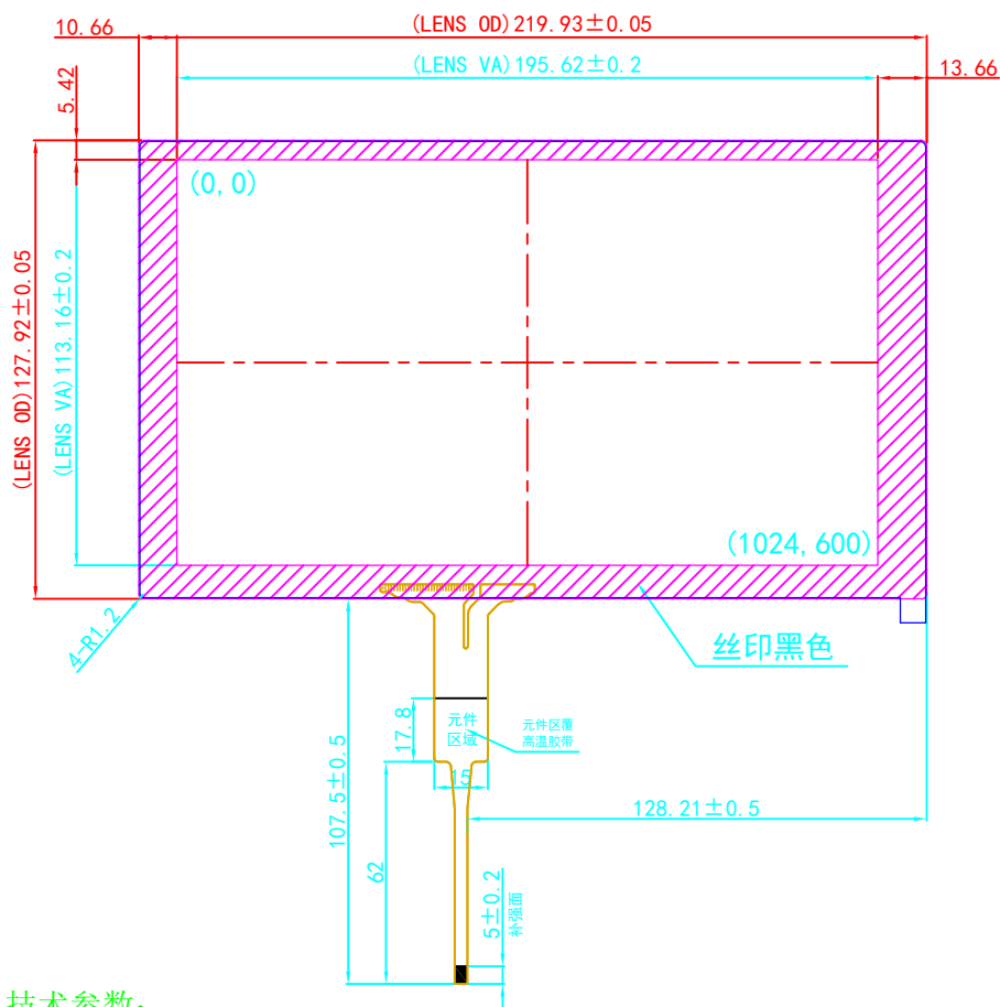
正视图
