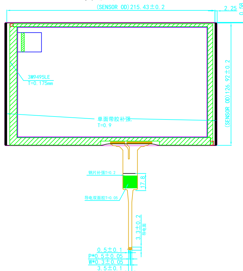
背视图
