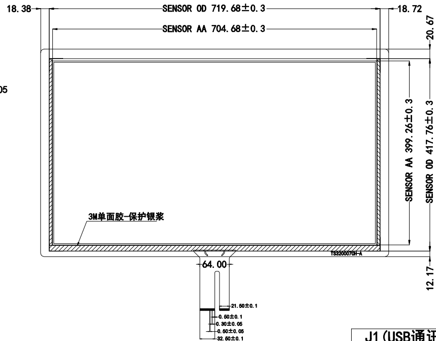
背视图
